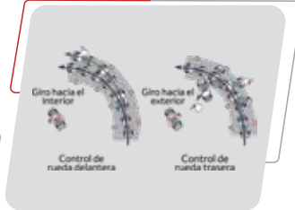
Sistema de control de estabilidad (VSC)
